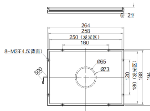
MV-MX-436-412-W
