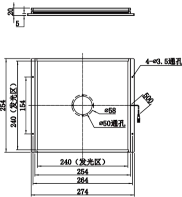
MV-MX-240-240-W
