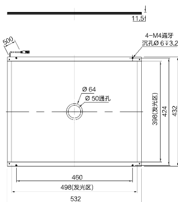
MV-MX-498-398-W2
