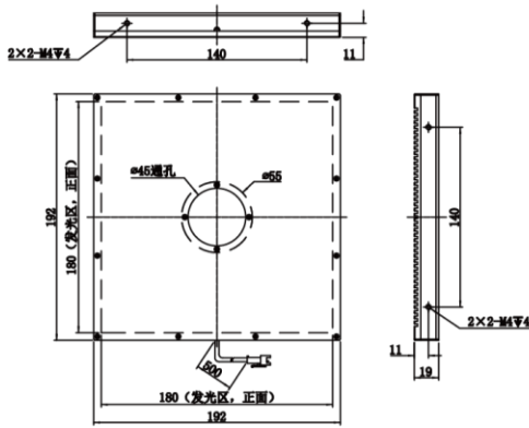
MV-MX-180-180-W/B
