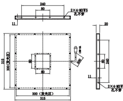
MV-MX-498-398-W2
