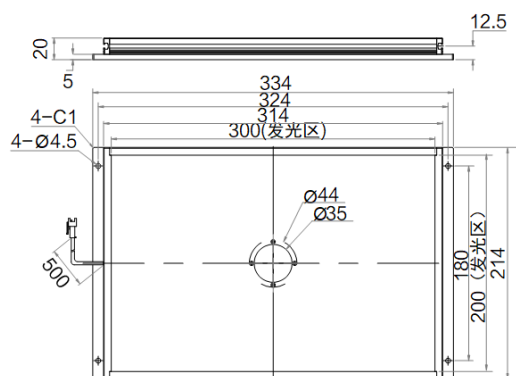
MV-MX-300-200-W
