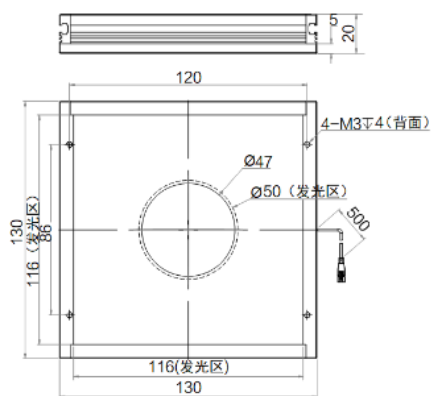
MV-MX-116-116-W
