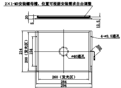
MV-MX-260-200-W
