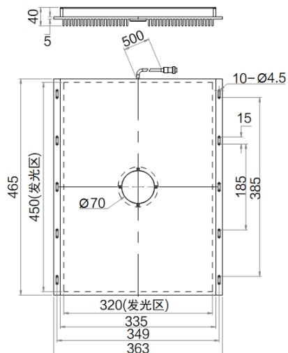
MV-MX-450-320-W2
