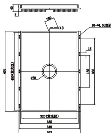
MV-MX-450-320-W
