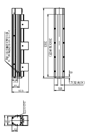
MV-LTHS-350-W
