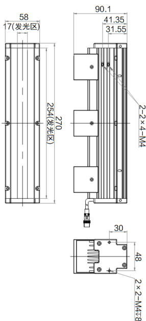
MV-LTHS-254-W
