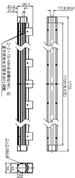
MV-LTHS-1700-W
