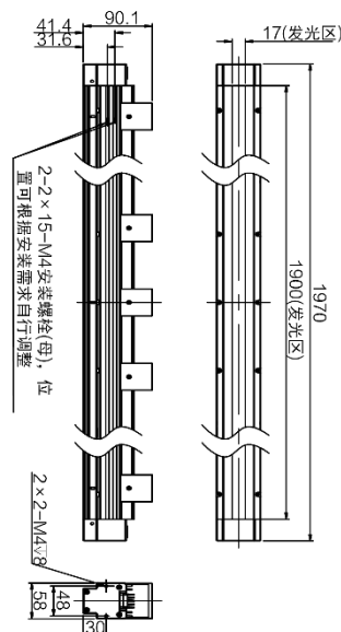
MV-LTHS-1900-W
