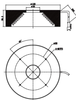
MV-LRM-120-45-W
