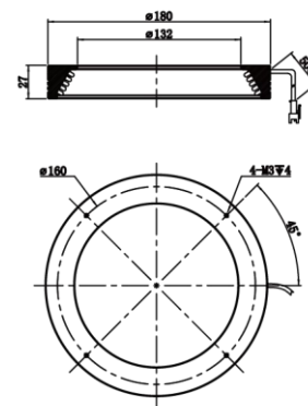
MV-LRM-180-30-W
