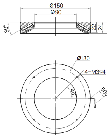
MV-LRM-150-60-W
