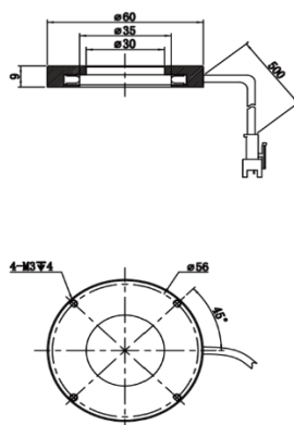
MV-LRM-60-0-R
