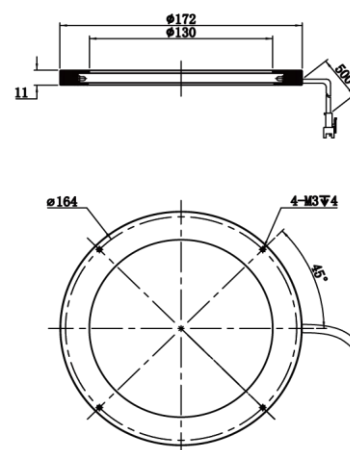
MV-LRM-172-0-W
