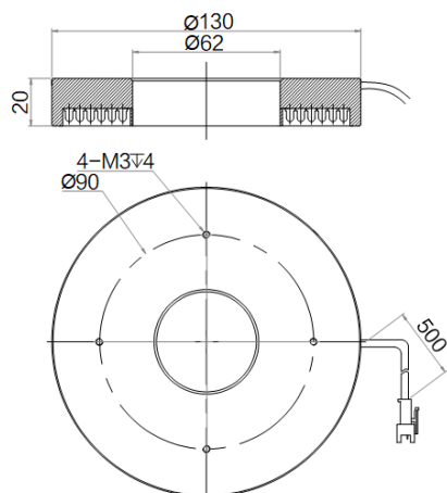
MV-LRM-130-90-R
