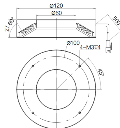
MV-LRM-213-30-W
