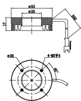
MV-LRM-53-90-W
