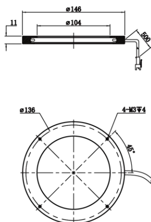
MV-LRM-146-0-W/IR940
