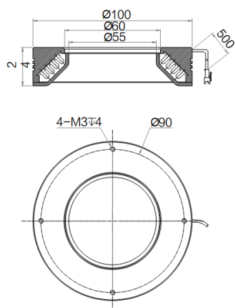
MV-LRM-100-45-W
