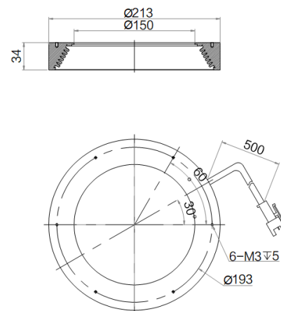
MV-LRM-213-30-W
