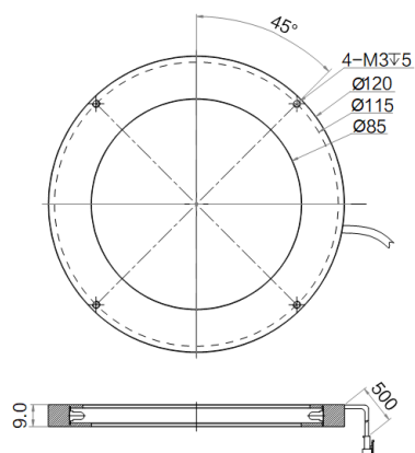
MV-LRM-120-0-WS
