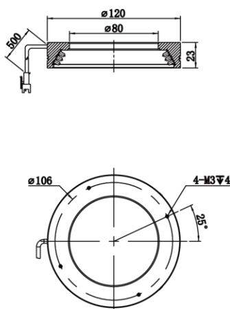
MV-LRM-120-30-W/B
