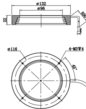
MV-LRM-132-20-W
