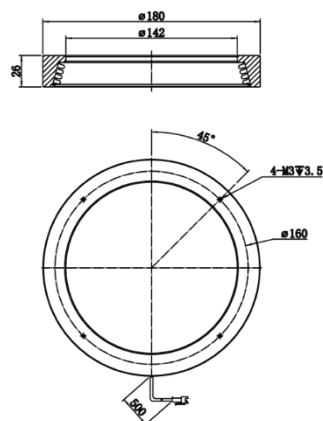
MV-LRM-180-15-W
