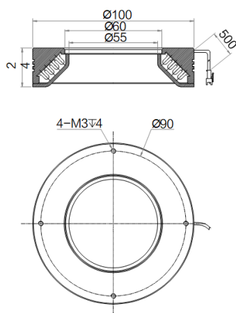
MV-LRM-100-45-W
