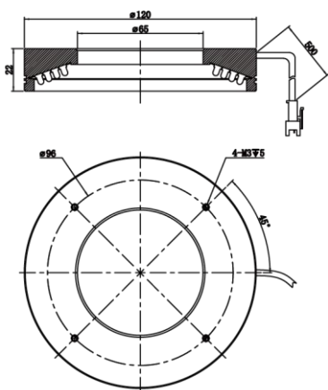
MV-LRM-120-70-W
