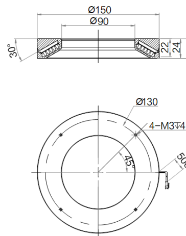
MV-LRM-150-60-W
