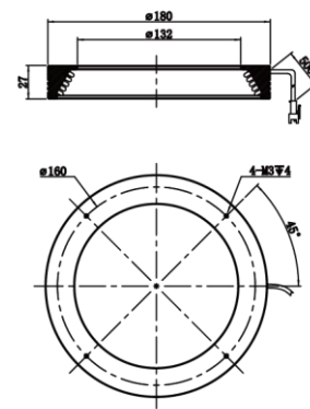
MV-LRM-180-30-W
