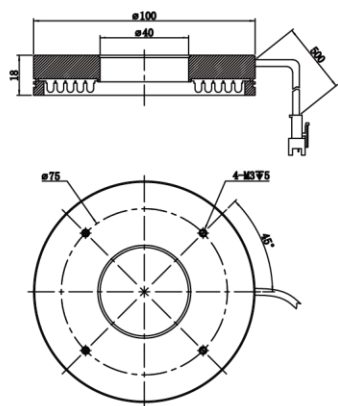
MV-LRM-100-90-W/R
