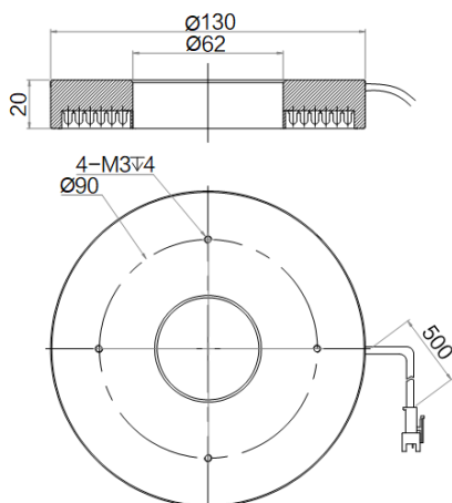
MV-LRM-130-90-R
