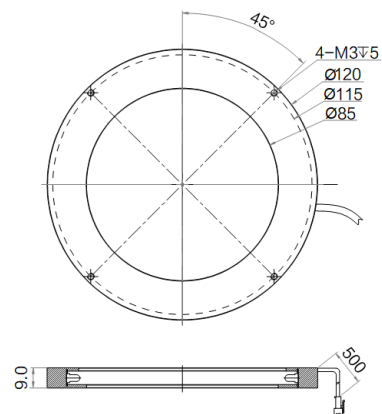
MV-LRM-120-0-WS
