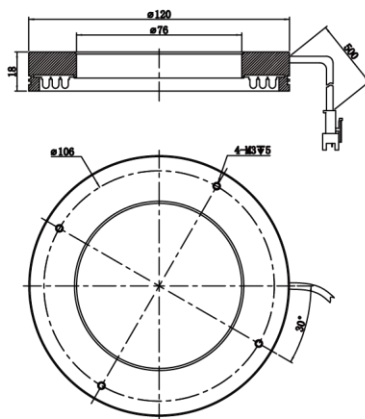
MV-LRM-120-90-W
