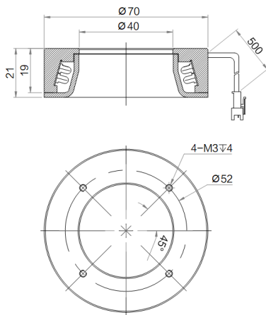
MV-LRM-70-15-W
