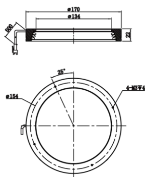
MV-LRM-170-20-W
