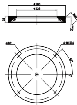
MV-LRM-180-60-W
