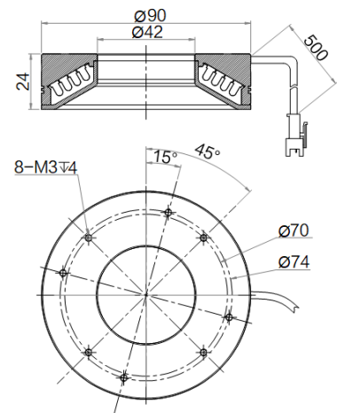
MV-LO-90-60-W
