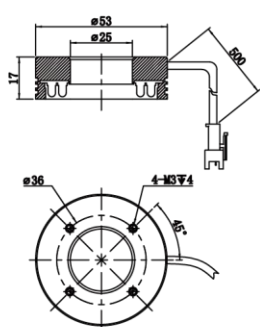
MV-LO-53-90-W
