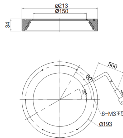
MV-LO-213-30-W
