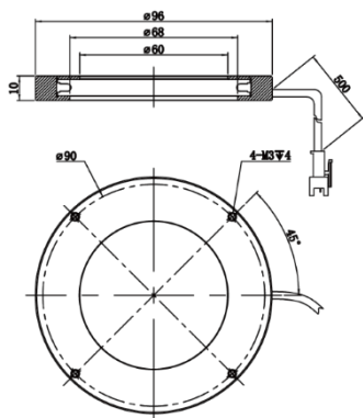
MV-LO-96-0-W/R
