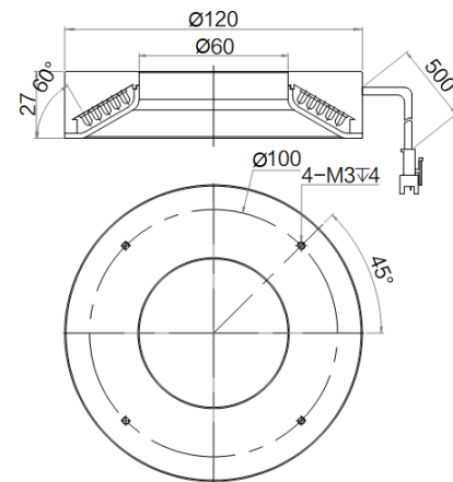
MV-LO-213-30-W
