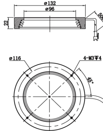
MV-LO-132-20-W
