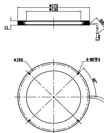
MV-LO-172-0-W
